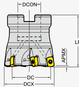
Cuerpo fresado
